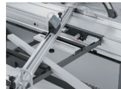
DIGIT L デジタル表示付き クロスカット・マイターフェンス 最大設定寸法3200mm
