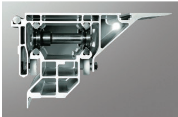
ダブルローラーキャリッジの断面
