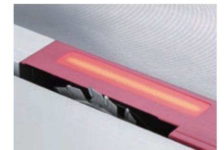
2軸制御スコアリング(ケビキ)軸 LEDスコアリング刃口付 水平、垂直位置微調整は電動式
