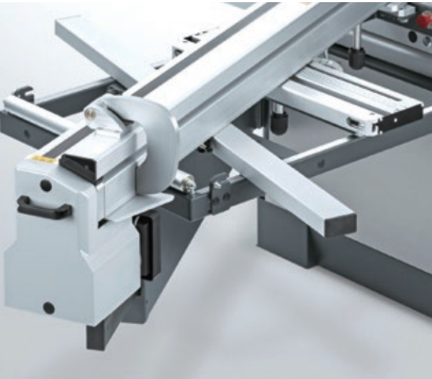
Duo Flex CNC × 2台 クロスカット・マイターフェンス
