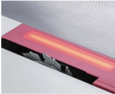
2軸制御スコアリング(ケビキ)軸 LEDスコアリング刃口付 0.75kw (1hp) 8200rpm (60Hz) 水平、垂直位置微調整は電動式 スコアリング軸作動時は安全のため刃口LEDが点灯 ※刃物はオプション
