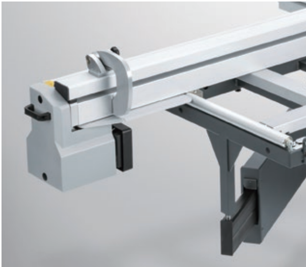
Duo 90 CNC × 2台 クロスカットフェンス
