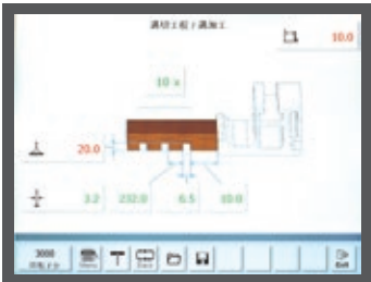
連続溝付メニュー
