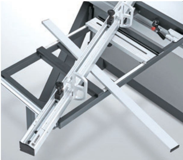
CMF クロスカット・マイターフェンス 長さ&角度アナログ表示
