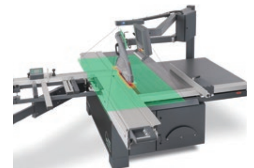
2台のカメラによる監視エリア
