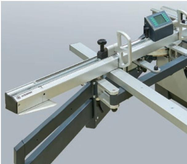
PQS LD パレログラム'クロスカット・マイターフェンス
