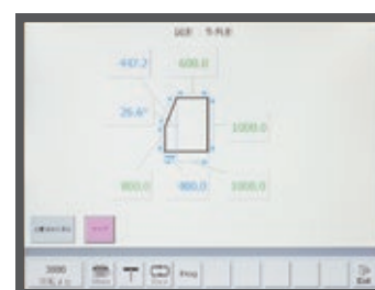
台形カットのカット寸法&角度計算
